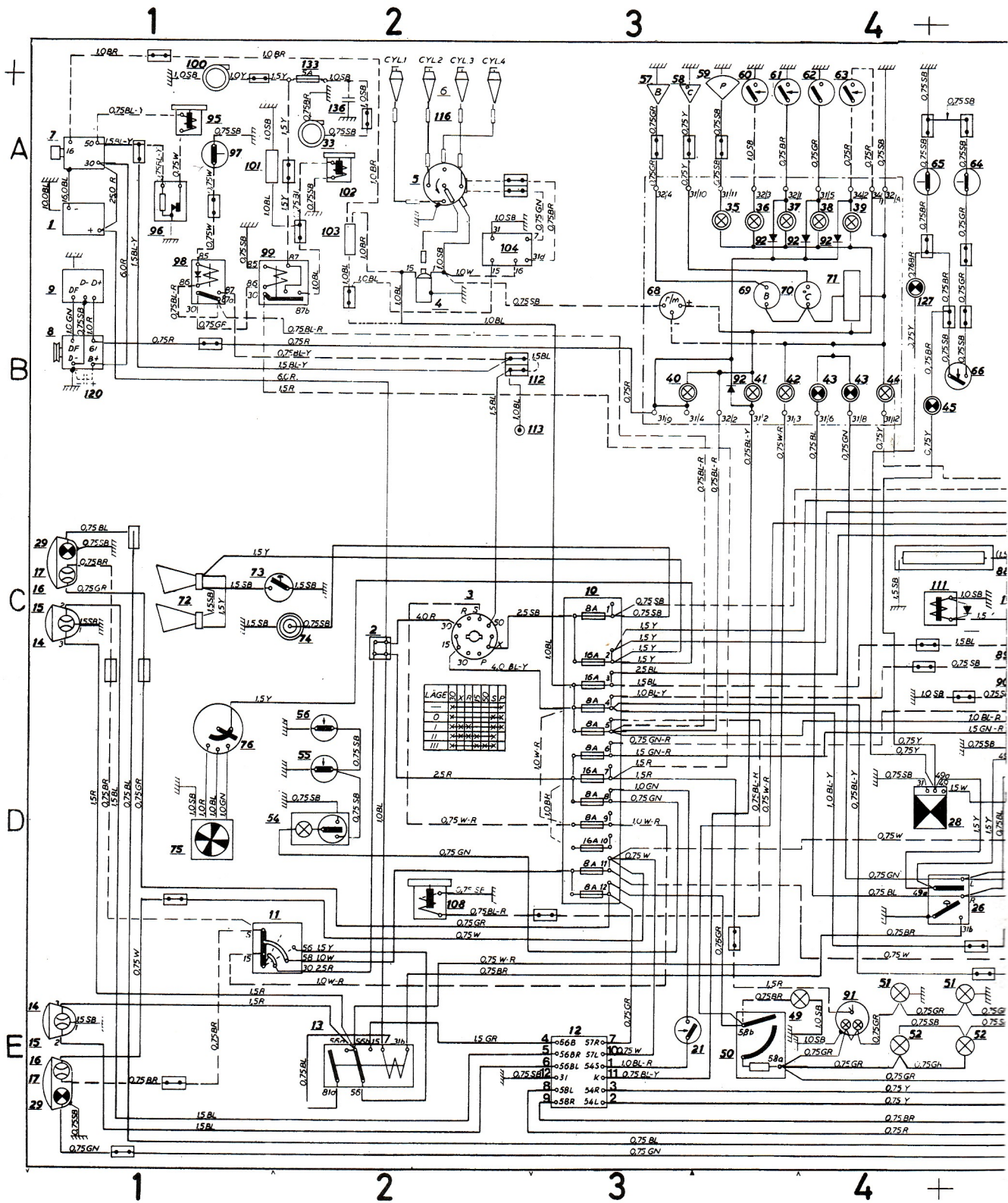
Kopplingschema för 1976 och 1977 års modeller
